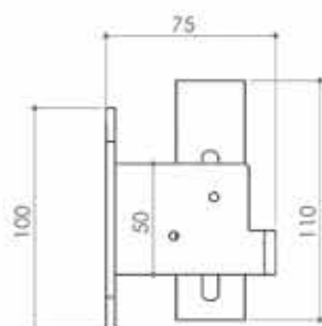
מתאם קיר
