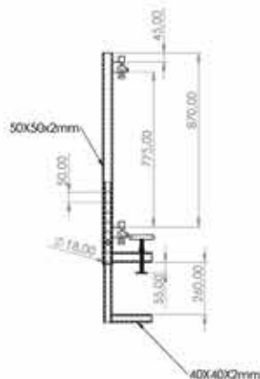
עמוד מלחציים צידי
