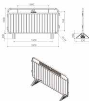
מחסום הולכי רגל מחוזק
