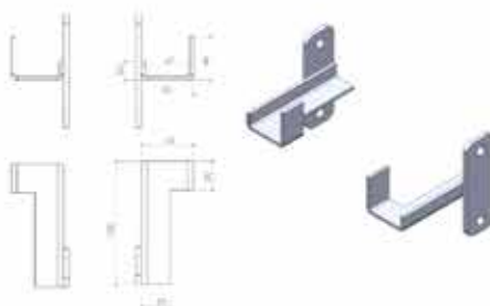
מתאם חיצוני
