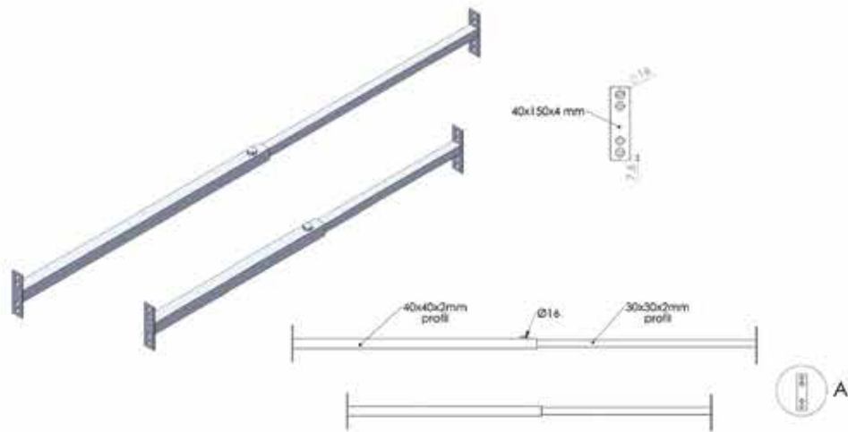
מעקה טלסקופי
